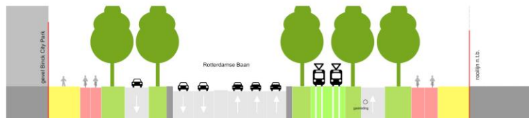
E - E'
